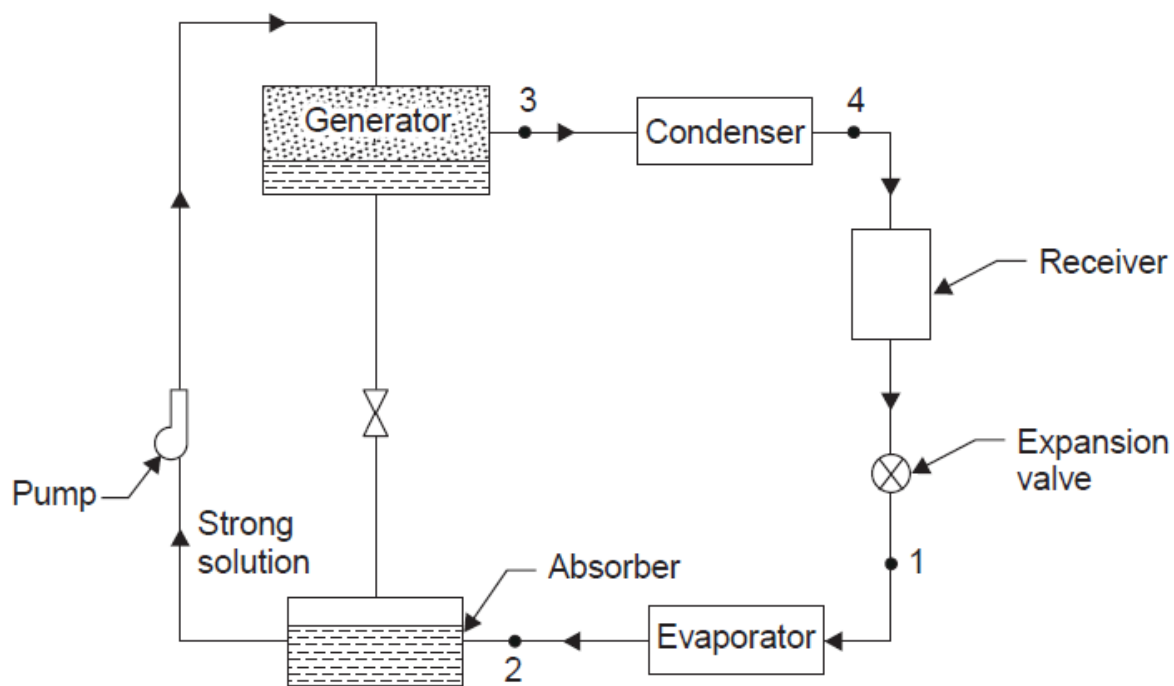
Simple vapour absorption system.
